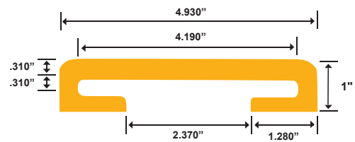
Redco™ Flange Cap Part #: R-32521
